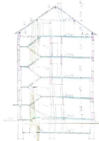
SCHNITT
