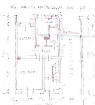
ERDGESCHOSS
