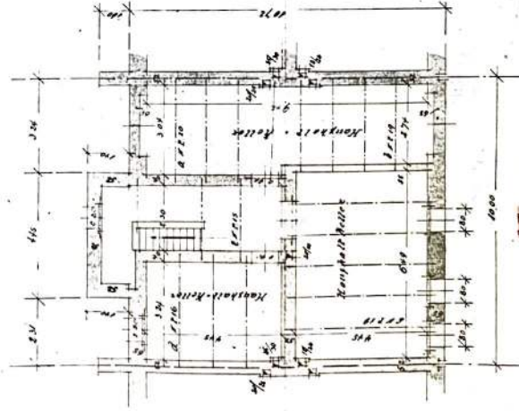
Kellerbachschoss
