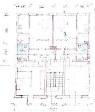
2.+3. OBERGESCHOSS
