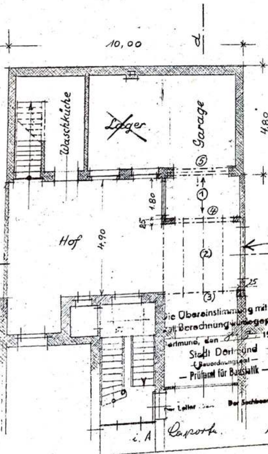
Erdgeschoss
