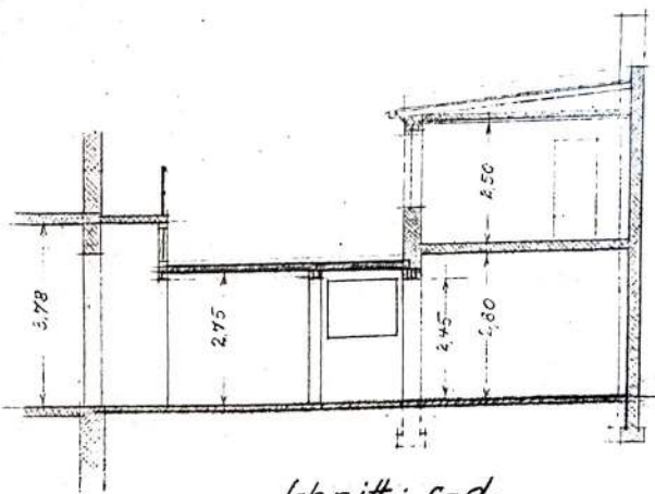
Schnitt: c-d
